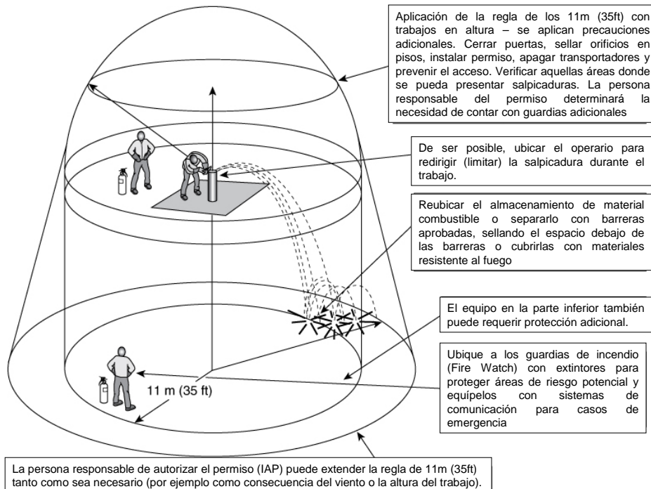
Ilustración de la utilización de múltiples guardias de incendio ( Fire Watch ) Fuente: NFPA 51B
